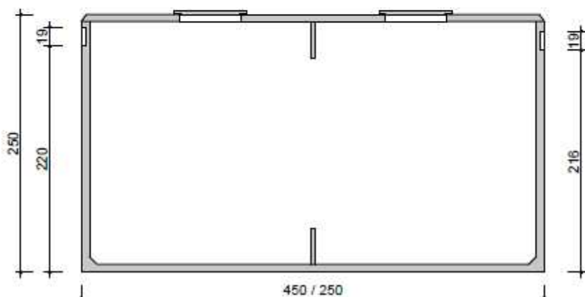
DOORSNEDE COUPE
