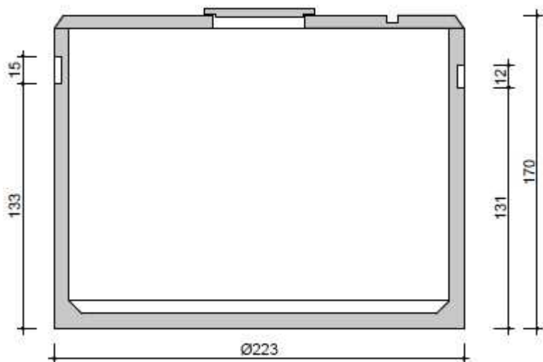
DOORSNEDE COUPE
