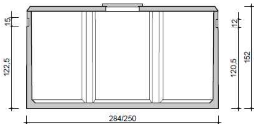
DOORSNEDE COUPE
